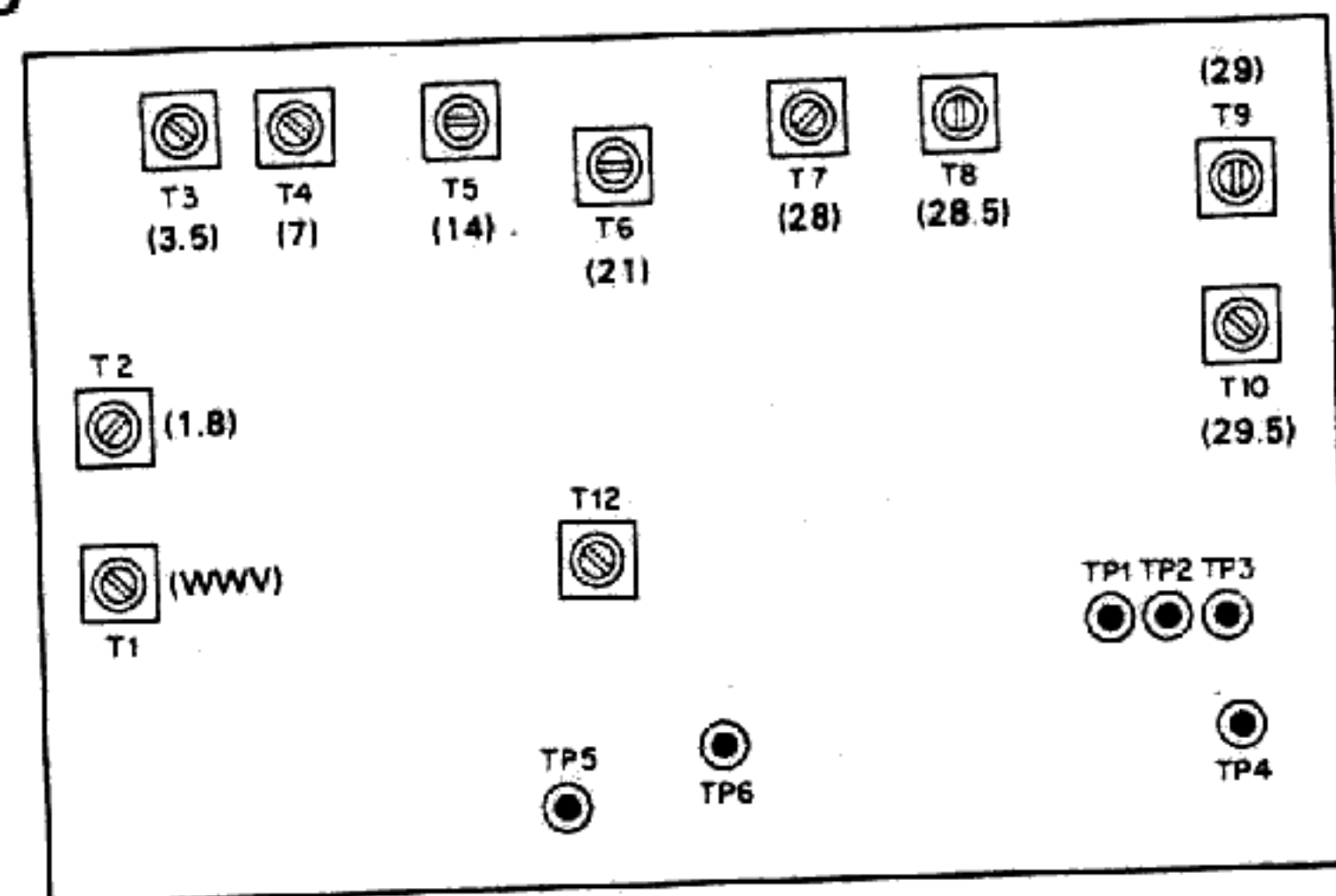
Fig. 22 VCO unit
